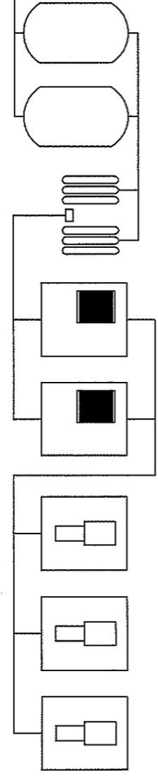
IMPIANTO ARIA COMPRESSA MEDICALE
